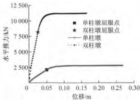
图 3 水平推力-位移关系对比
